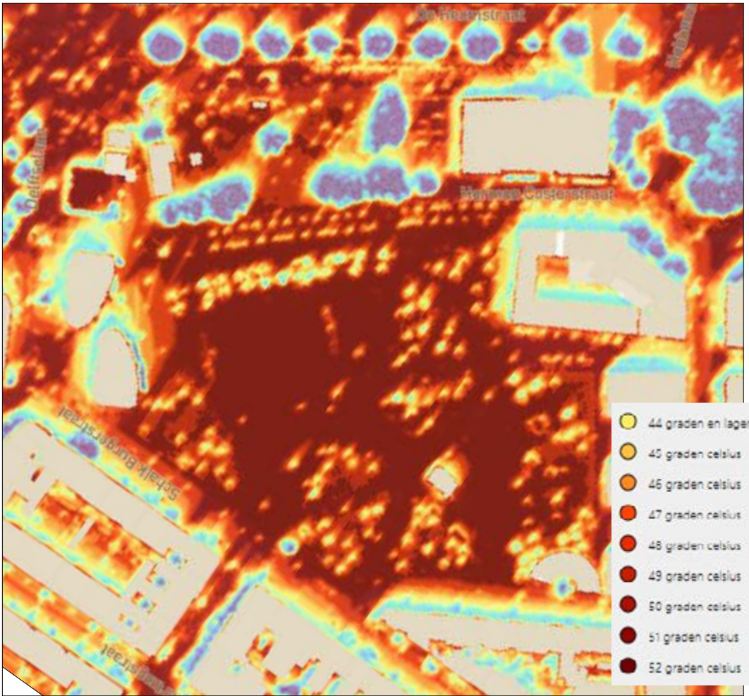
Gevoelstemperatuur
